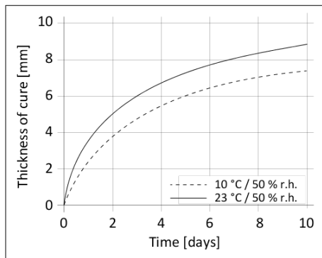
Diagramm 1: Sikaflex®-292i kuivamise kiirus
